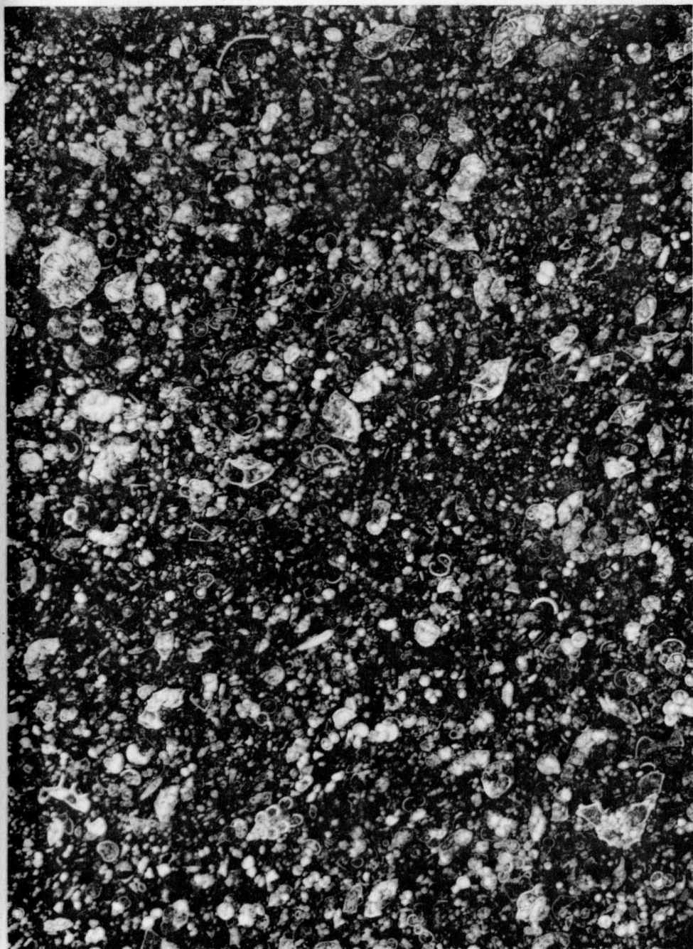
Fig. 4. Scaglia con prevalente Globotruncana stuarti (DE LAPP.) = Zona 1b''.
