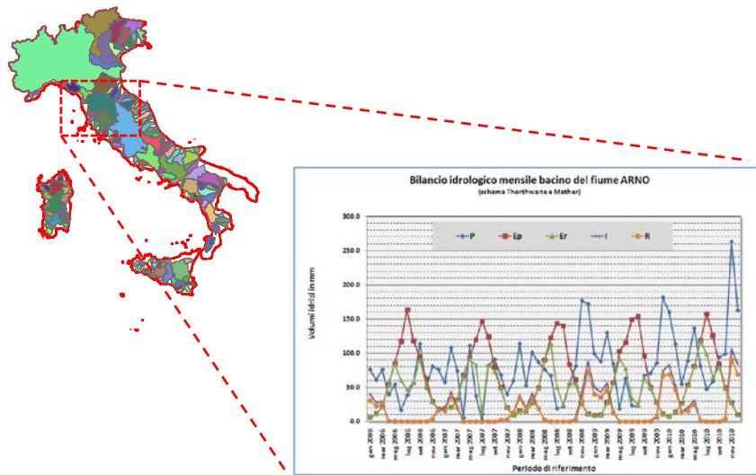
Figura 3: Esempio di bilancio idrologico mensile per il bacino idrografico del fiume Arno 7
