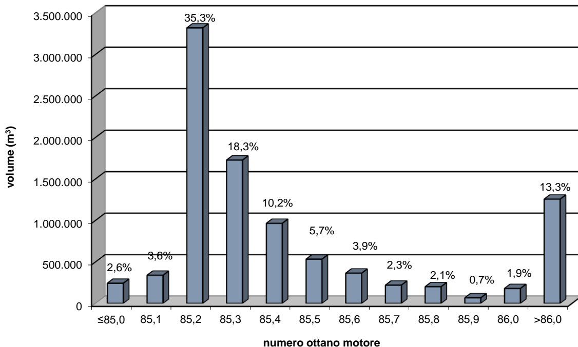
Fig. 5 Distribuzione del volume di benzina commercializzata nell'anno 2021 in funzione del numero di ottano motore
