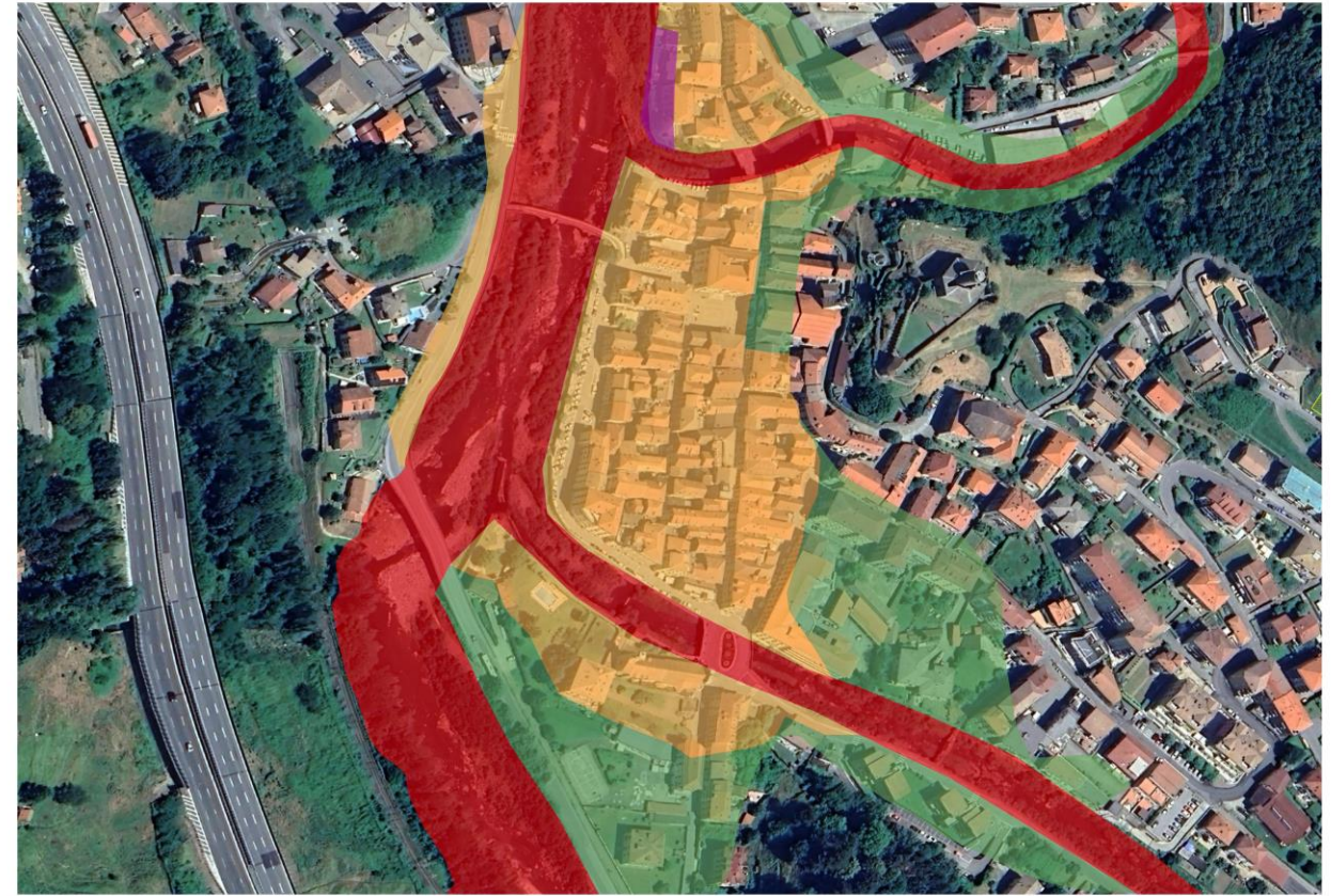
FASCE FLUVIALI POST INTERVENTI
