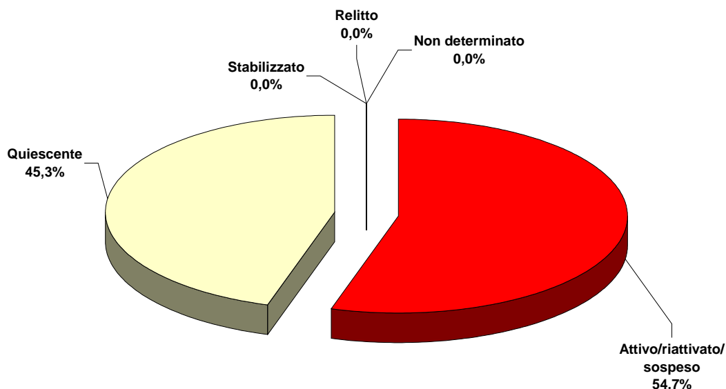
Figura 13.13 Percentuale delle frane per stato di attività (numero dei fenomeni).
