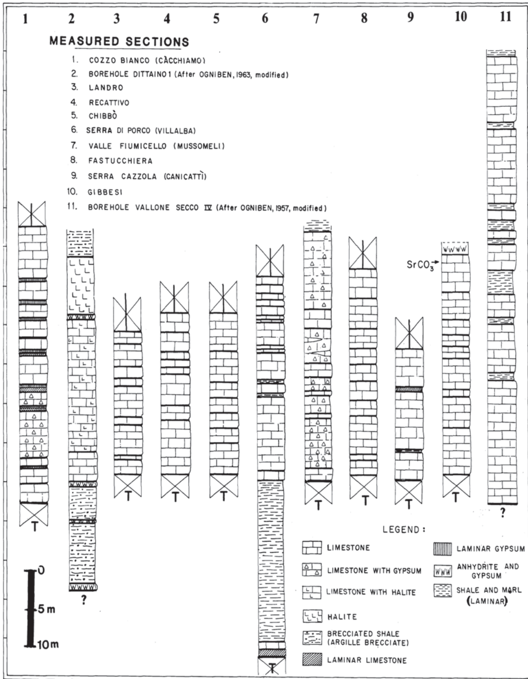
Le sezioni, misurate nel Calcere di Base, sono allineate secondo la base della formazione. T = Tortoniano superiore-Messiniano inferiore e marne e/o diatomi.
