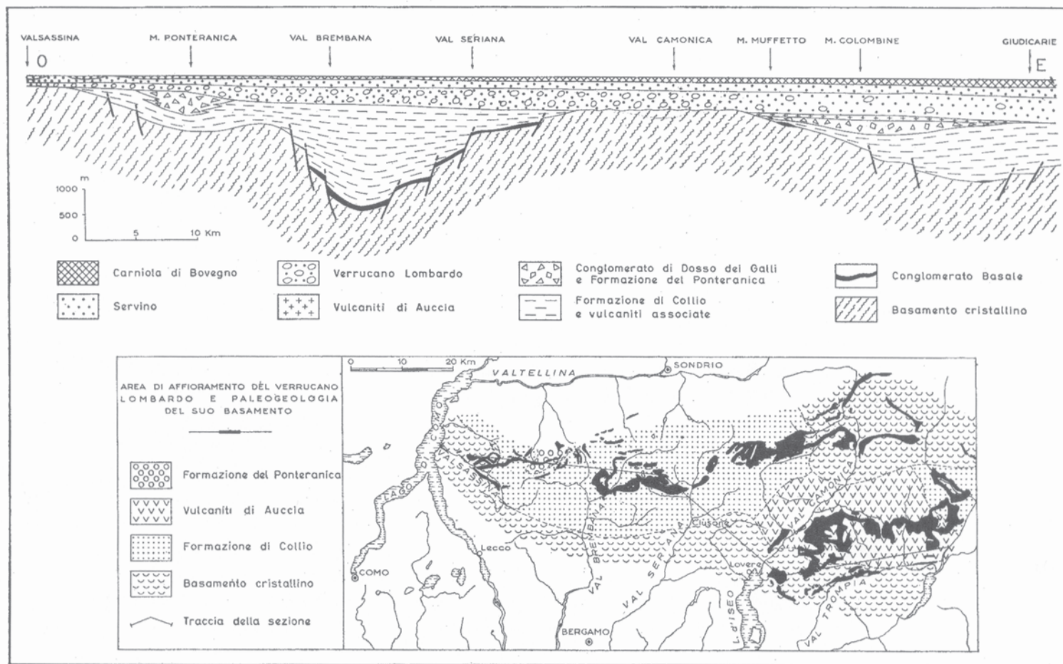
Area di affioramento del Verrucano Lombardo e sezione O-E lungo le Alpi Meridionali.
